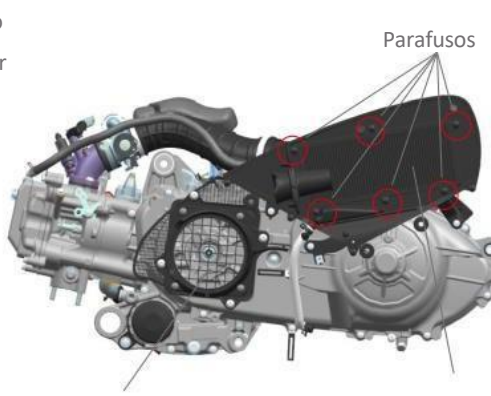
Filtro de ar
