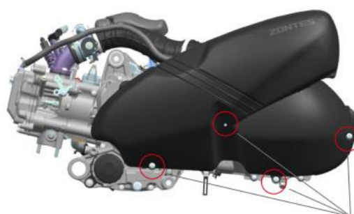
M6X 16 Parafusos de cabeça sextavada
